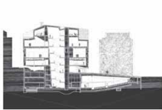
Пресек кроз трг и објекат © Herzog & de Meuron
